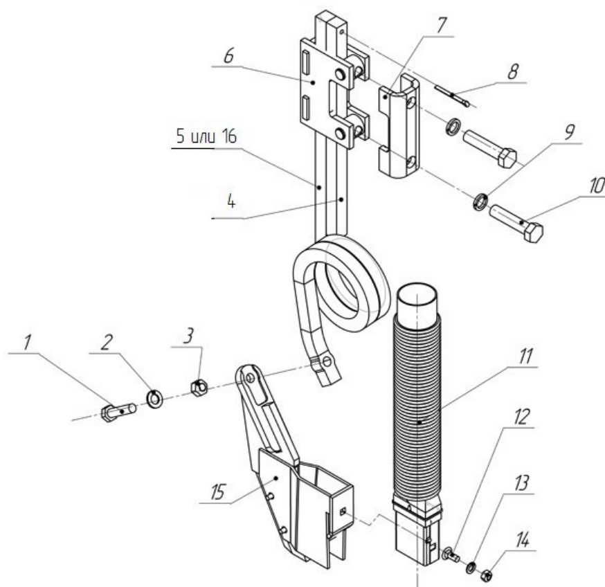
509.046.9170 Туковый сошник (правый)
