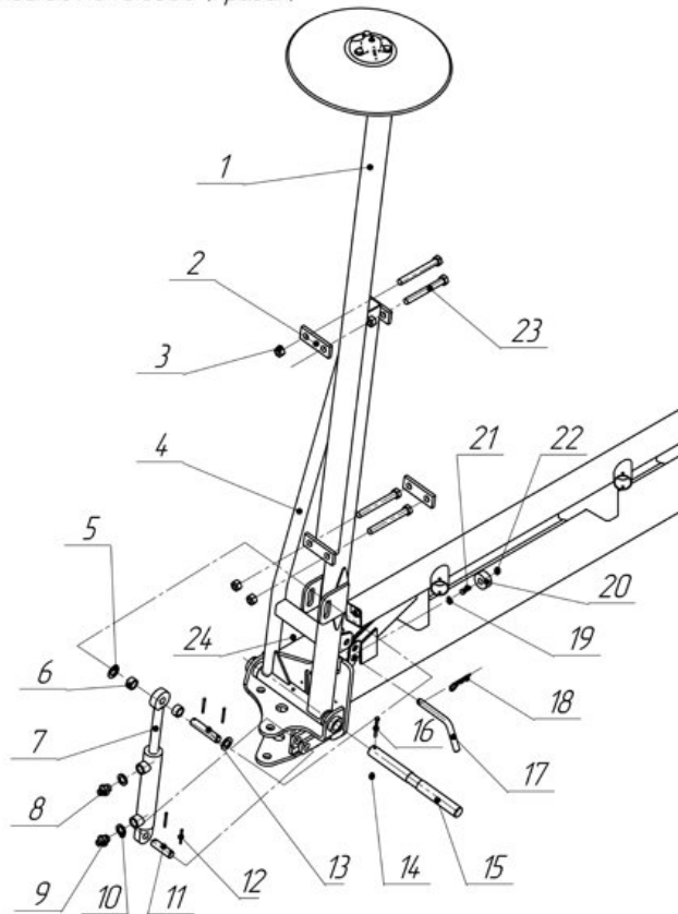
Штанга 509.046.8360 (правая)
